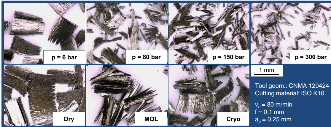
Fig. 14. Chip morphology.
