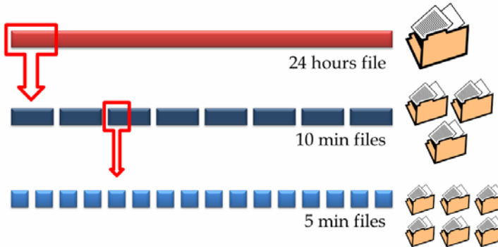
Fig. 14. Data files split schema
