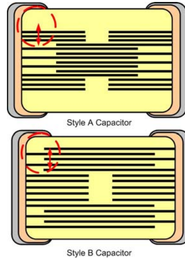
Fig. 2. 'Standard' vs. 'ESD-Enhanced' 0603 MLCC
