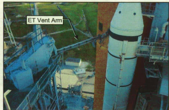
Figure 9. ET H2 Vent Arm
