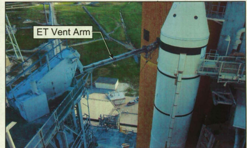
ET H2 Vent Arm
