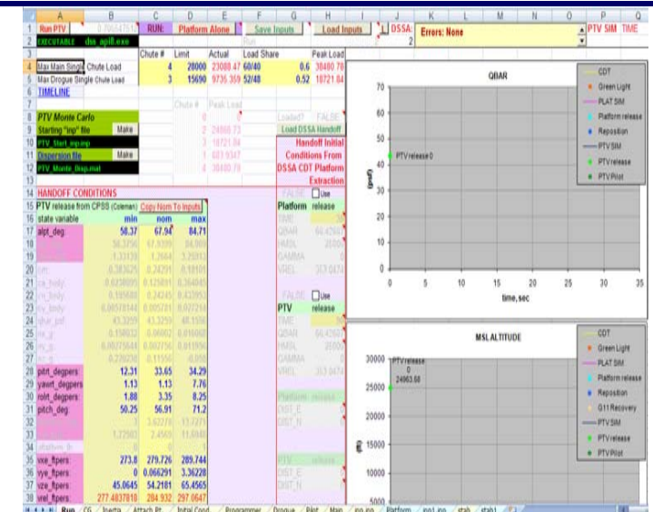
CAPSIM GUI
