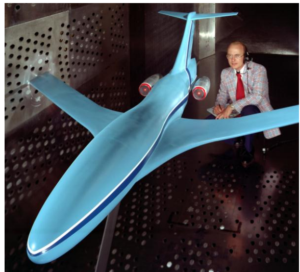
Figure 5. ATT wind tunnel model. 3
