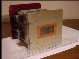
Rcv Array / Boeing 20 GHz (ICAPA)
