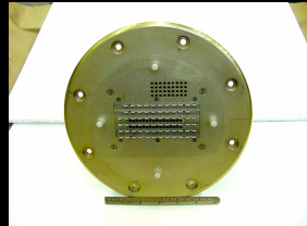
Rcv/Xmt Array AATT/WINCOM Ku-Band / Boeing
