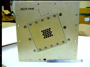
Rcv Array / Boeing 20 GHz (MASCOM)
