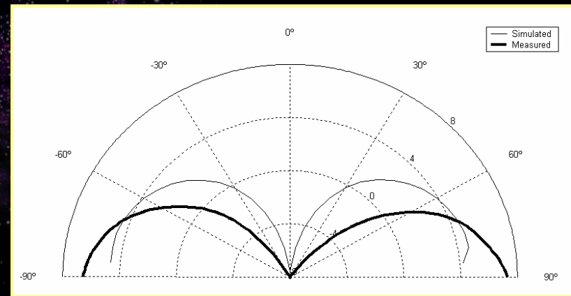
H-plane Pattern
