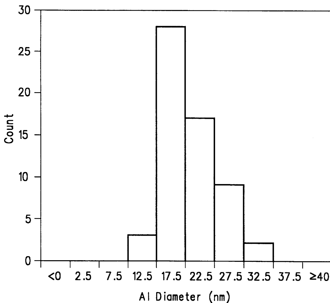
Al-7 at. % Y-5 at. % Fe Melt Spun Ribbon Anneal 275°C, 10 minutes
