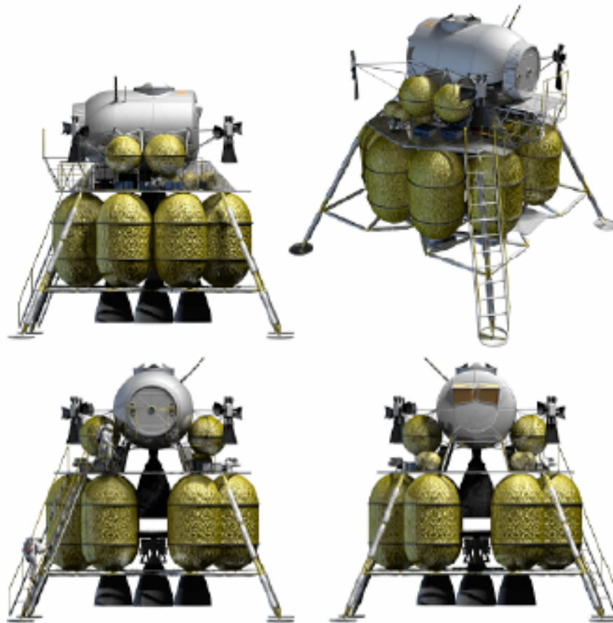
Figure 2. ESAS Lunar Surface Access Module.
