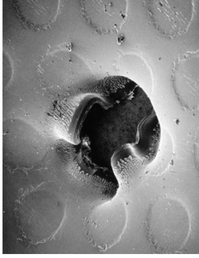
STS-90 Radiator
