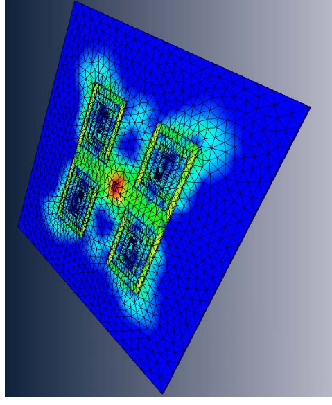
EIGER Simulation
