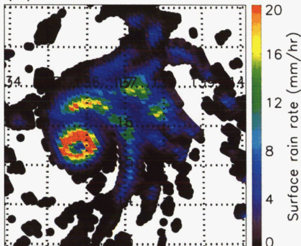
(d) BAYESIAN-MEAN
