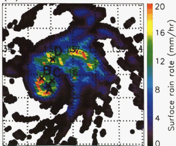
(d) BAYESIAN-MEAN
