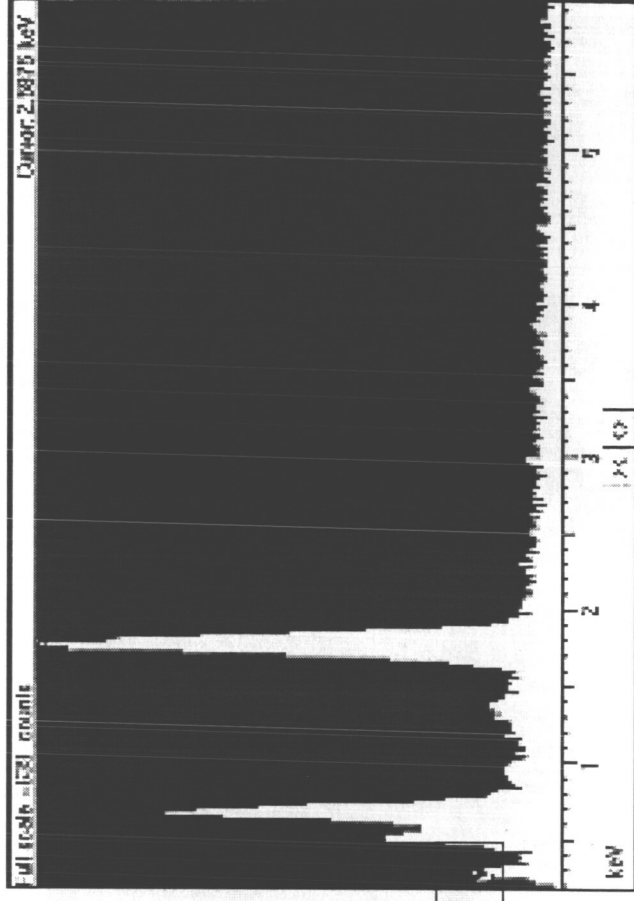
EDS Spectrum
