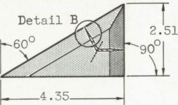
Fin F; fin area, 5.46; aspect ratio, 2.31.
