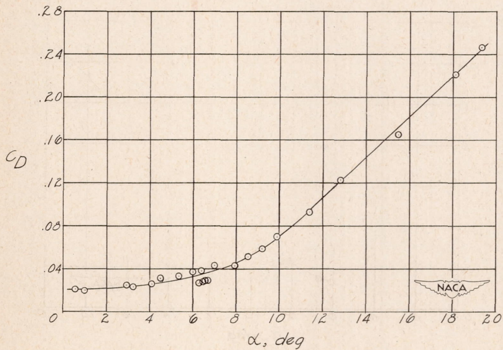
(d) M = 0.80 .
