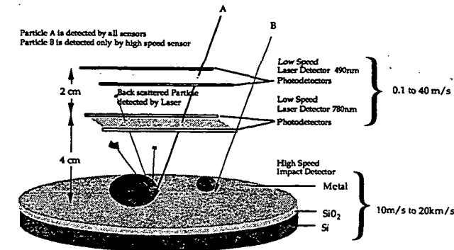
Fig 1. UPDE sensor.
