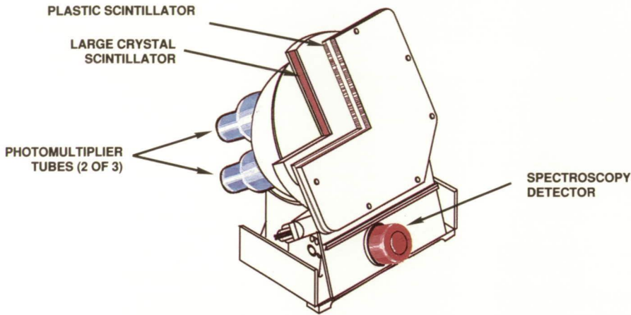
BATSE detector module
