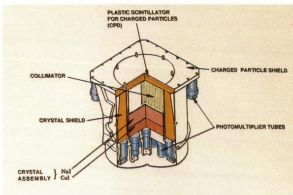
OSSE detector module (1 of 4)
