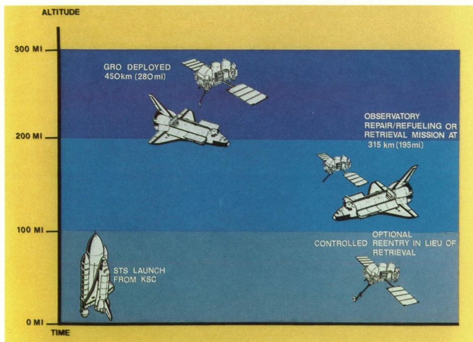
GRO mission scenario
