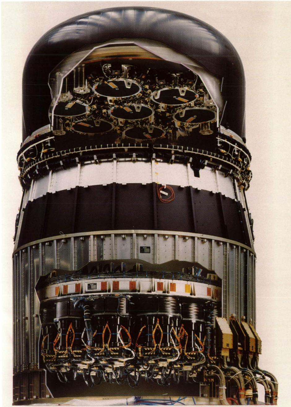
COMPTEL
