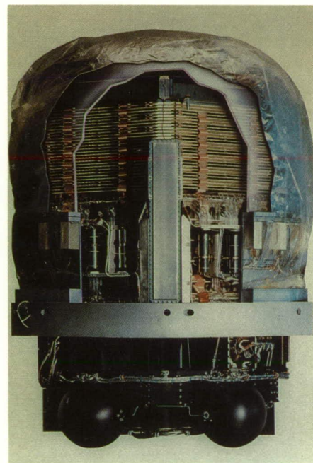
EGRET
