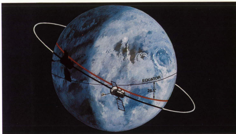
GRO orbit
