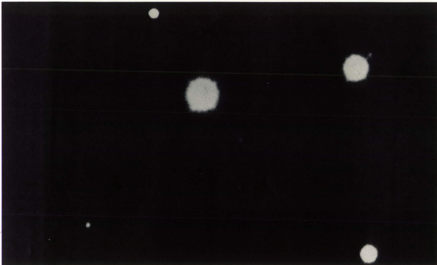
Quasar 3C 273
