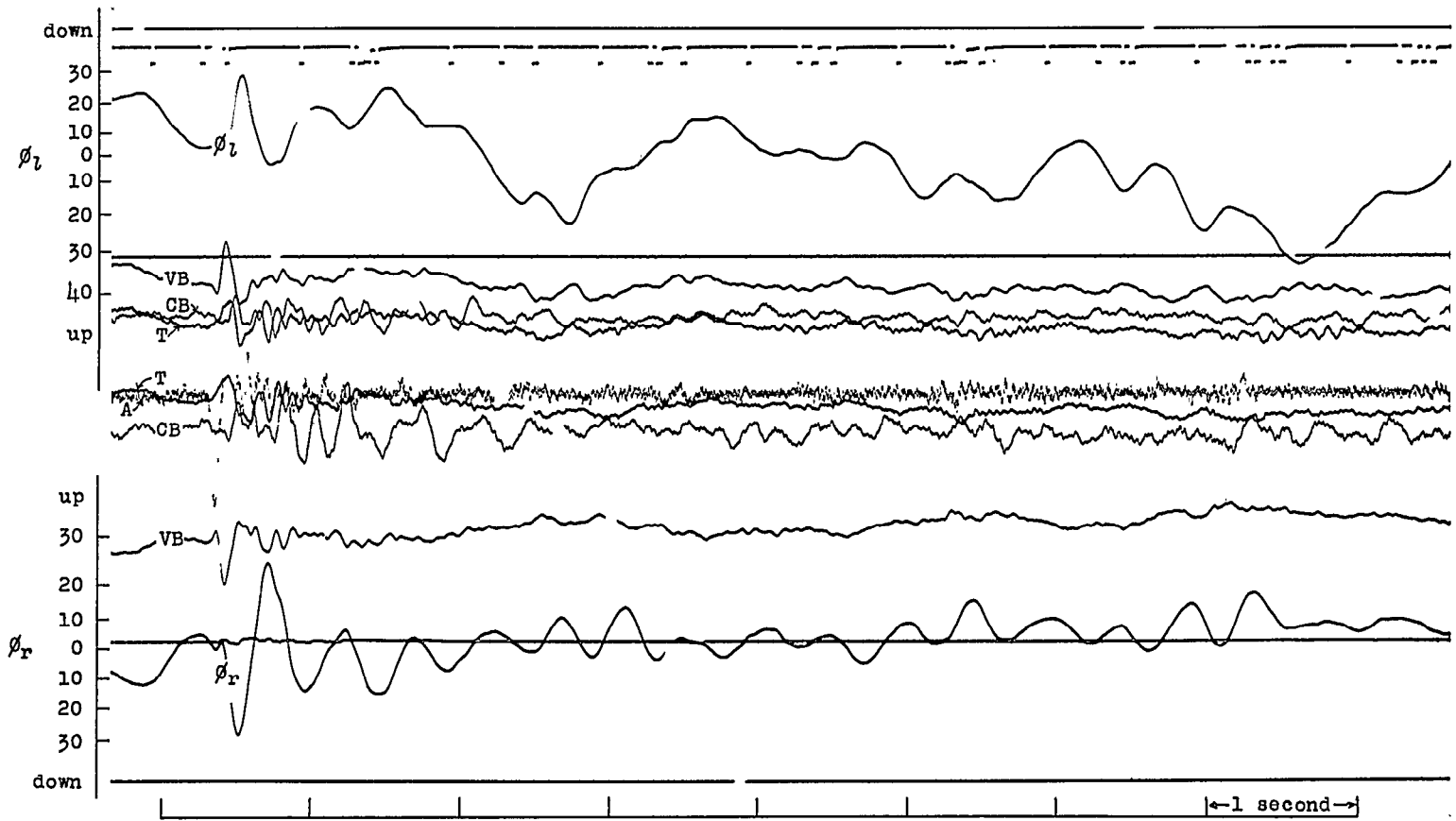
(d) V = 102.8 mph; symmetric excitation.
