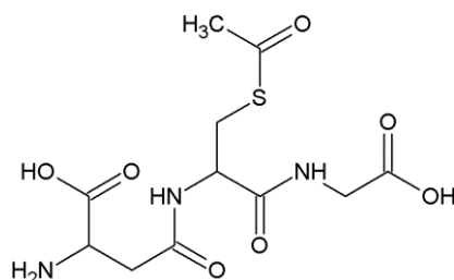
Fig. 9. S-acetylglutathione (SAG)
