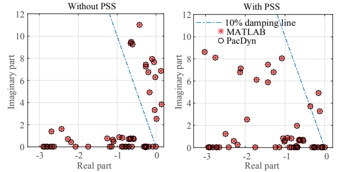
Fig. 15 – 68-bus system: Plots of eigenvalues
