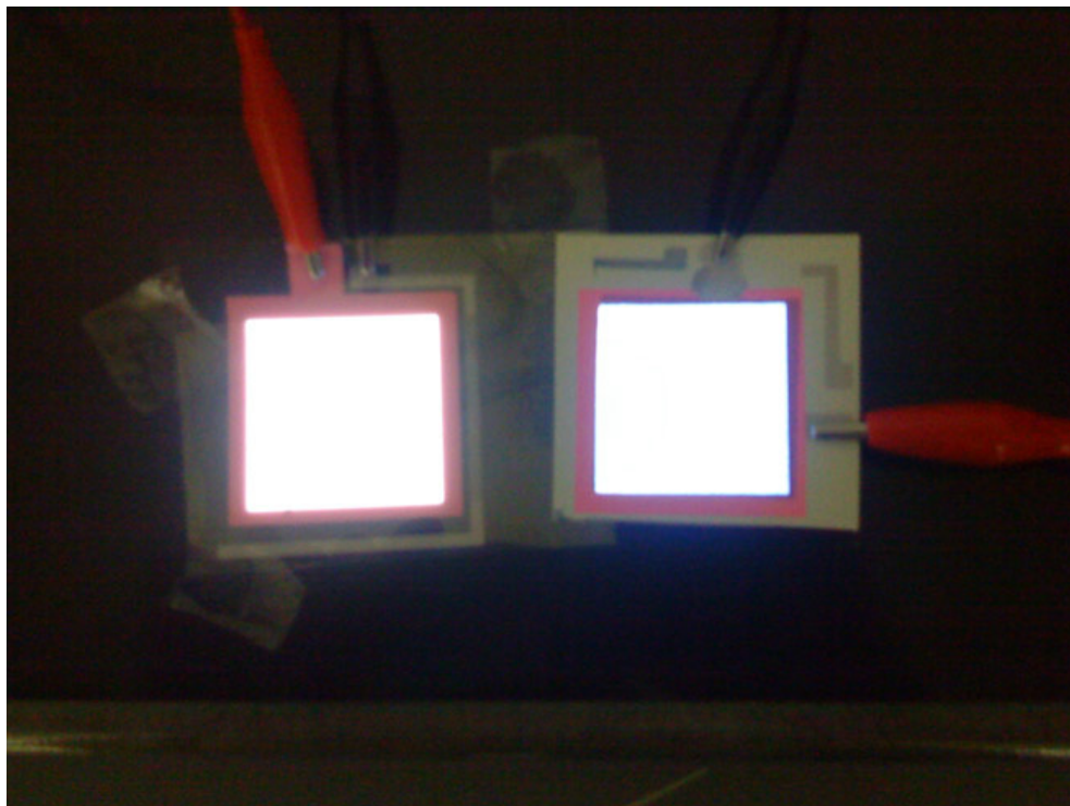
Ffigwr 3(b): Cymhariaeth weledol o'r lampau electroymoleuol a gynhyrchwyd drwy ddefnyddio ITO (ar y chwith) a PEDOT:PSS ar bapur (ar y dde) fel yr electrod tryloyw
