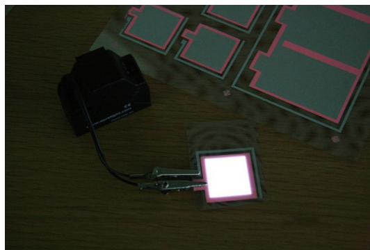
Ffigwr 2: Creu'r lampau drwy ddefnyddio peiriant printio sgriniau. Dangosir y dull o wneudlampau ar ITO. Ar bapur mae'r drefn yn wahanol, gyda haen ychwanegol o PEDOT:PSS ar ben y ffosfor.
