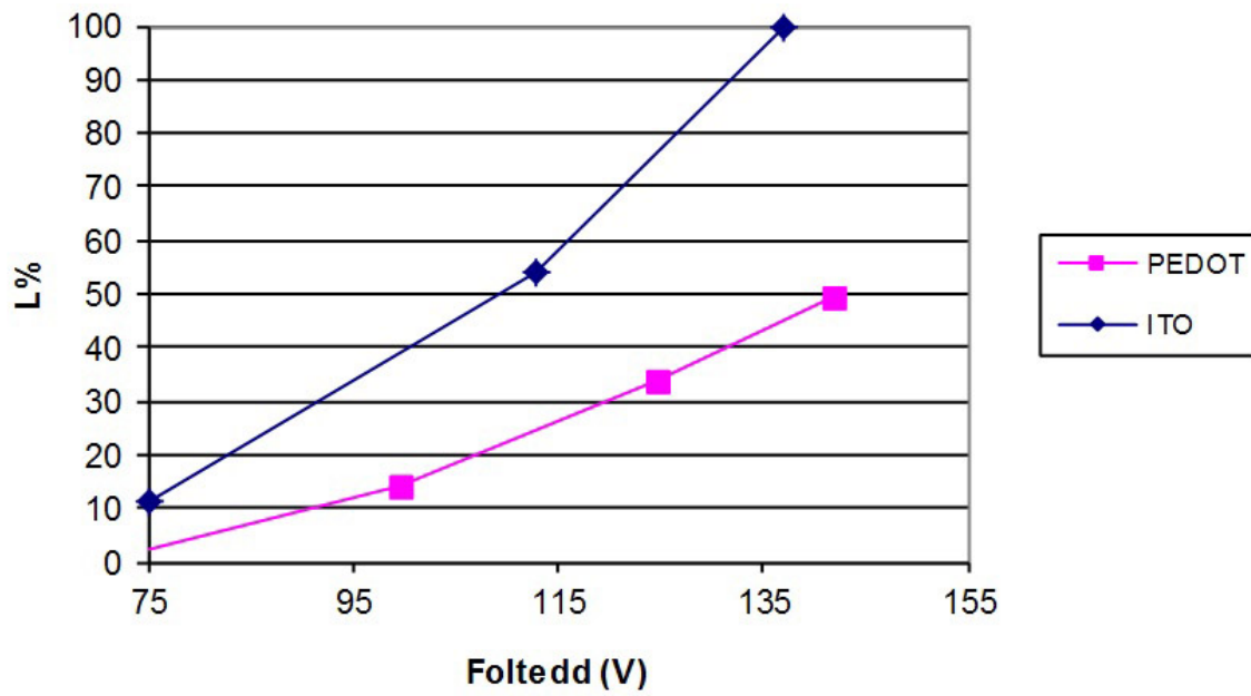
Ffigwr 3(a): Perfformiad lampau electroymoleuol a gynhyrchwyd drwy ddefnyddio PEDOT:PSS ac ITO fel yr electrod tryloyw
