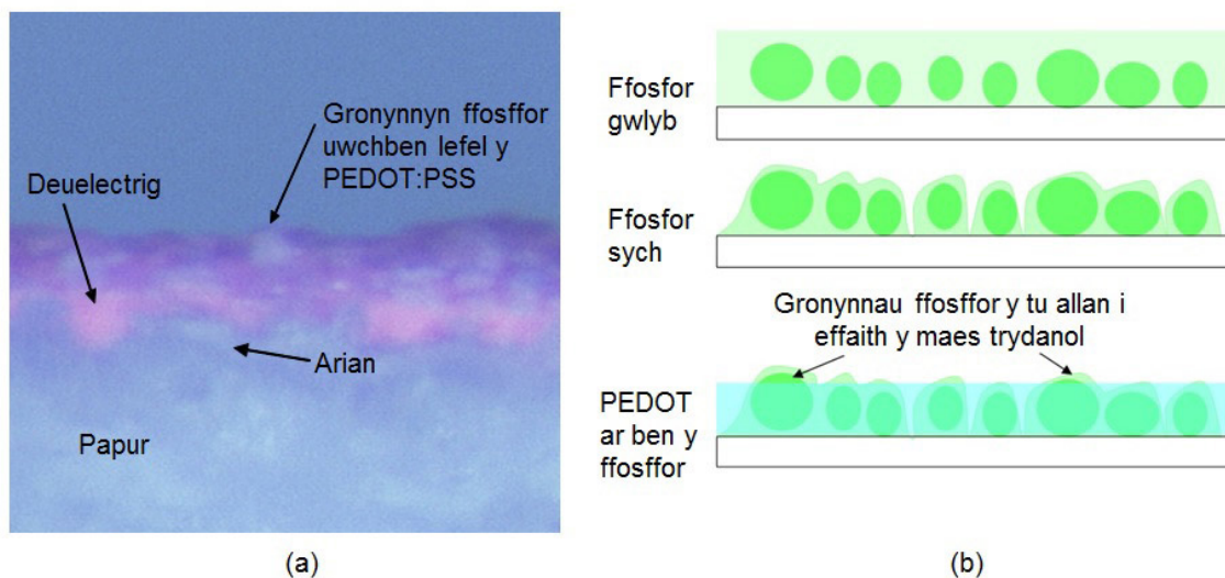
Ffigwr 8(a): Trawstoriad drwy'r lamp ar bapur, a (b) darlun sgematig o'r hyn sy'n achosi lleihad yn nysgleirdeb y lampau. Yn (b) mae'r gronynnau ffosfor y tu allan i effaith y maes trydanol.
