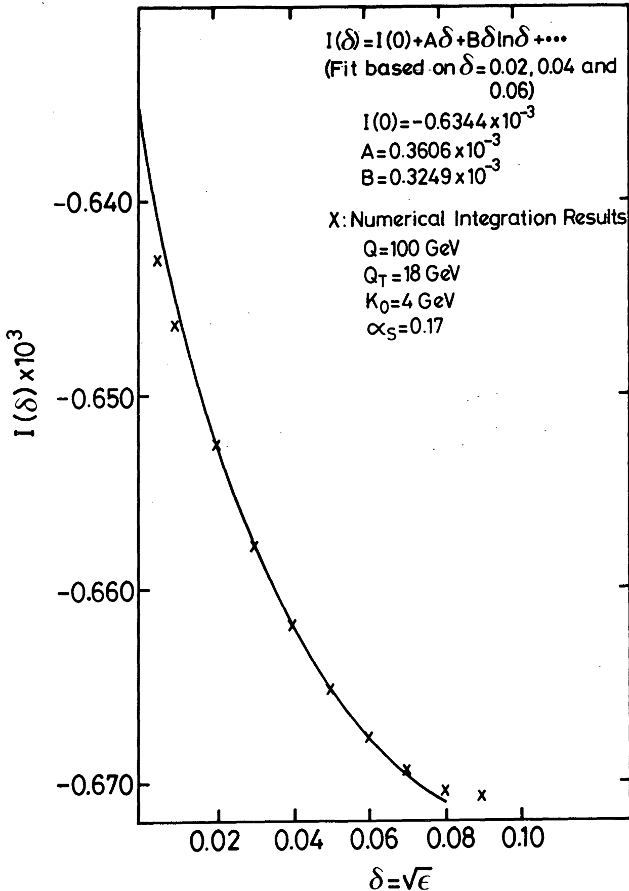
Figure V.2.3 : \epsilon -extrapolation
