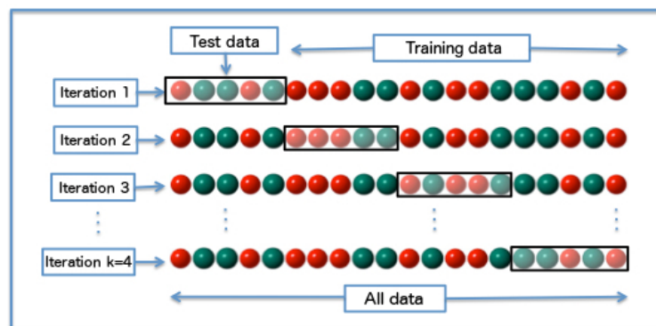
ABBILDUNG 4.2: 4-fold Cross validation (Quelle: http://bit.ly/2nB7IDW )
