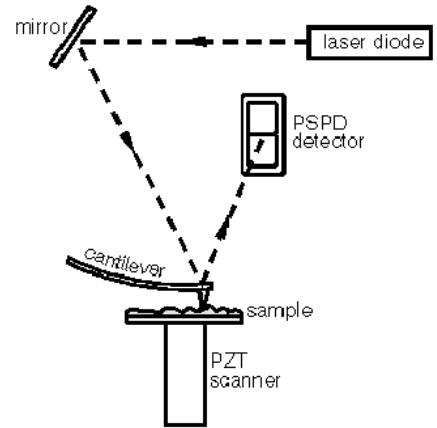
图 3 下扫描方式扫描力显微镜
