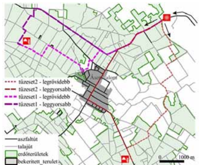
4. ÁBRA: HÁLÓZATELEMZÉSSEL KIJELÖLT LEGRÖVIDEBB ÉS LEGGYORSABB ÚTVONALAK KÉT ELKÉPZELT TŰZESETHÉZ A SZEGED FELŐL ÉRKEZŐ TŰZOLTÓAUTÓK SZÁMÁRA
