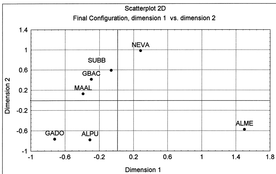
FIG. 3. Análisis MDS aplicado a los datos de presencia/ausencia para cada especie por unidades corológicas.
