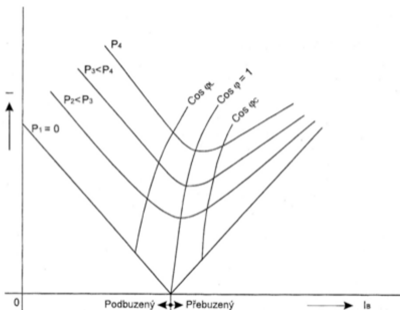
Obr. 4.1 V-křivky synchronního stroje [2]
