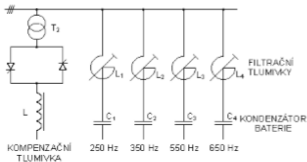
Obr. 4.8 Plynulé řízení kompenzace
