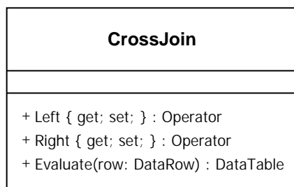
Obrázek 11: Diagram třídy CrossJoin
