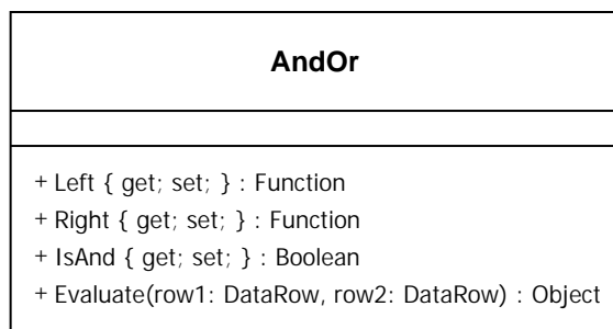
Obrázek 23: Diagram třídy AndOr
