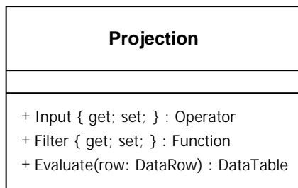
Obrázek 7: Diagram třídy Projection
