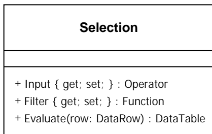
Obrázek 6: Diagram třídy Selection
