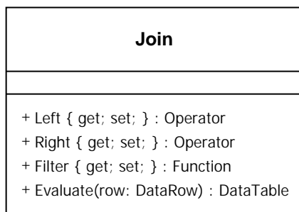
Obrázek 9: Diagram třídy Join
