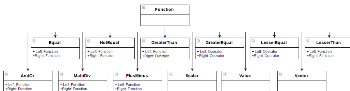
Obrázek 4: Třídní diagram funkcí
