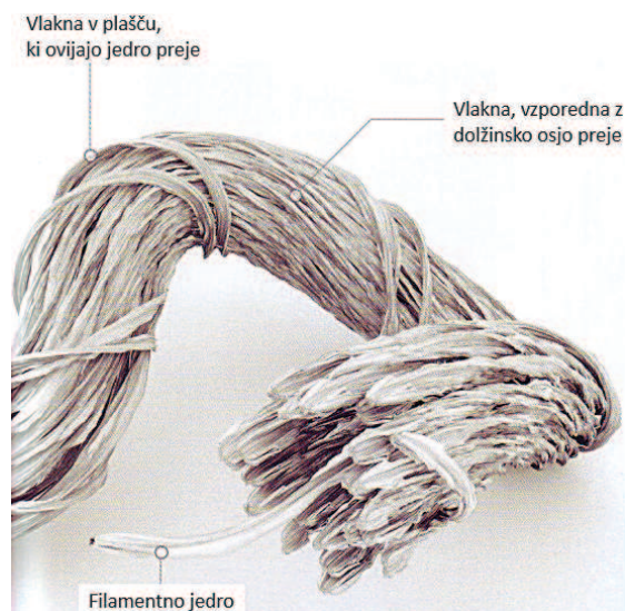
Slika 6: Struktura preje, izdelane na predilniku Corizon [6]
