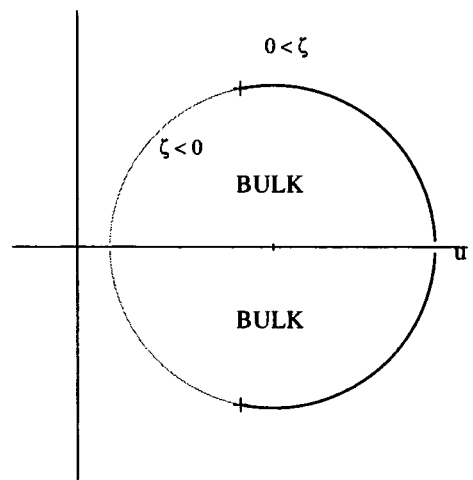
(d) Supercritical brane
