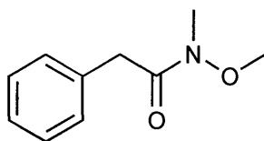
148
