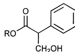
202 143
