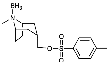
164
