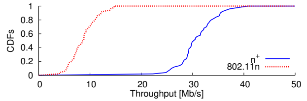
(d) Throughput of tx3-rx3
