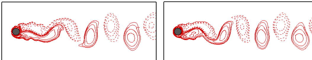
(e) St_f = 0.7
