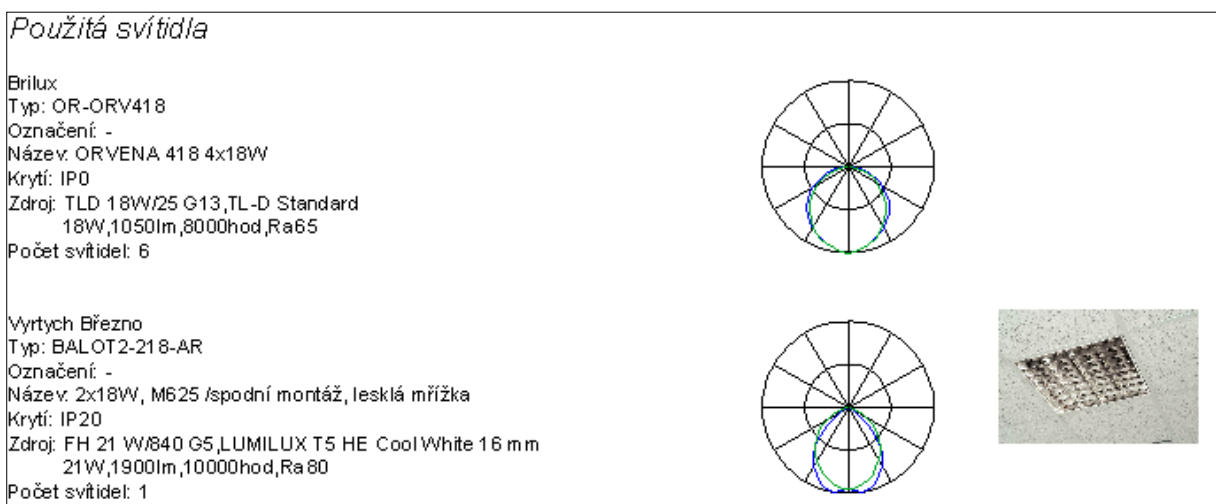
Obr. 12: Použitá svítidla
