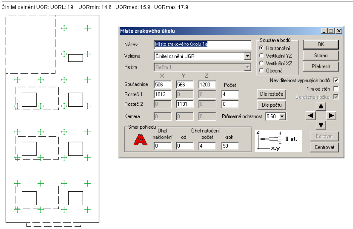
Obr. 11: Nastavení UGR
