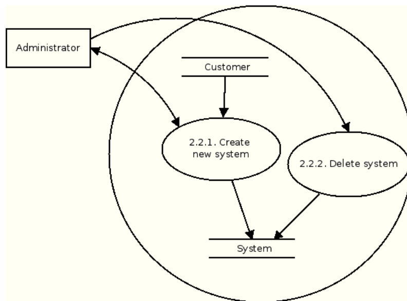
Obrázek 9: DFD diagram úrovně 2 - správa systémů
