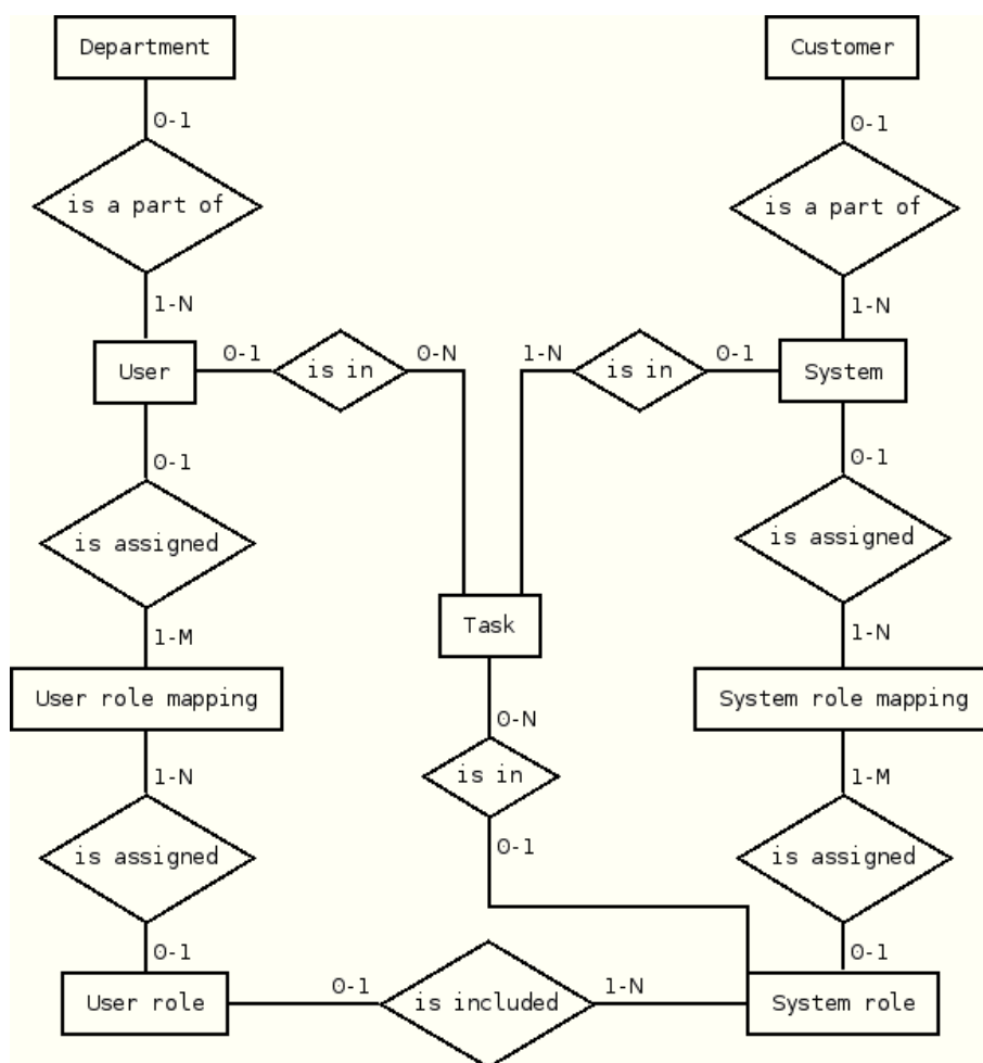
Obrázek 2: ER diagram
