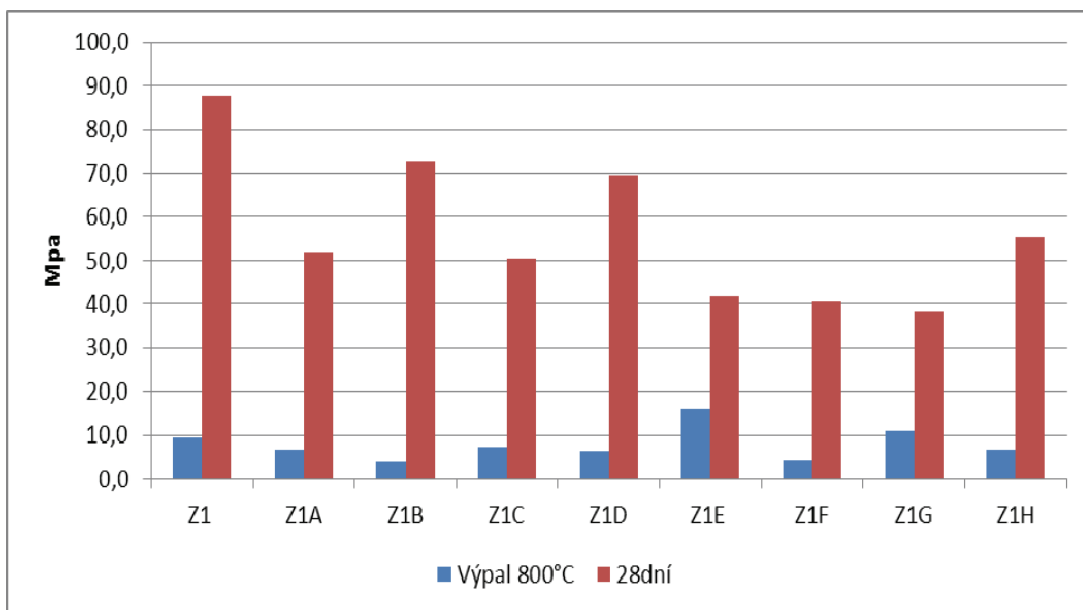
Obr. 5: Pevnost v tlaku po vystavení teplotě 800°C v porovnání s pevností po 28 dnech
