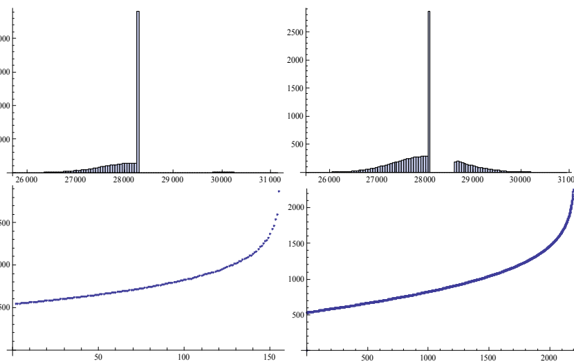
Obrázek 6 Histogram pravděpodobnostního rozdělení a průběh ztráty pro k = 0.9 (vlevo) a k = 0.25 (vpravo).
