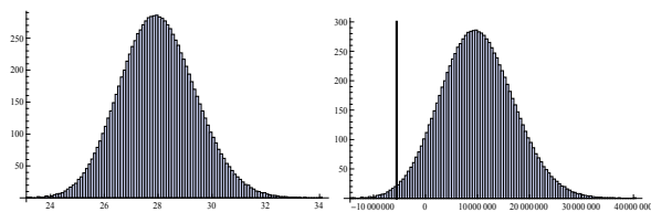
Obrázek 1 Histogram pravděpodobnostního rozdělení konečného kurzu (vlevo) a zisku (vpravo)
