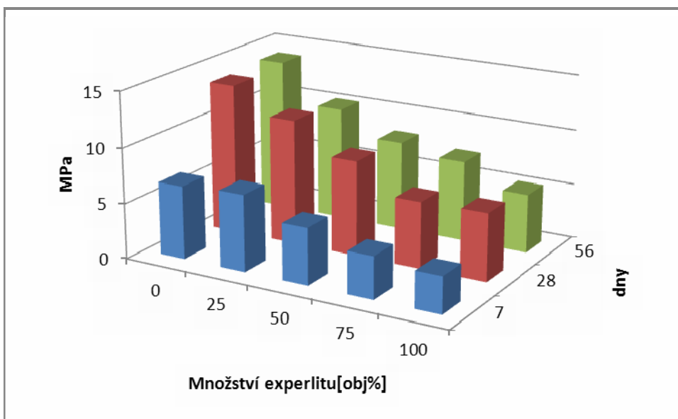
Obr. 3: Vývoj pevnosti v tlaku v závislosti na čase a množství použitého experlitu u lehkých malt s metakaolínem N-META 2
