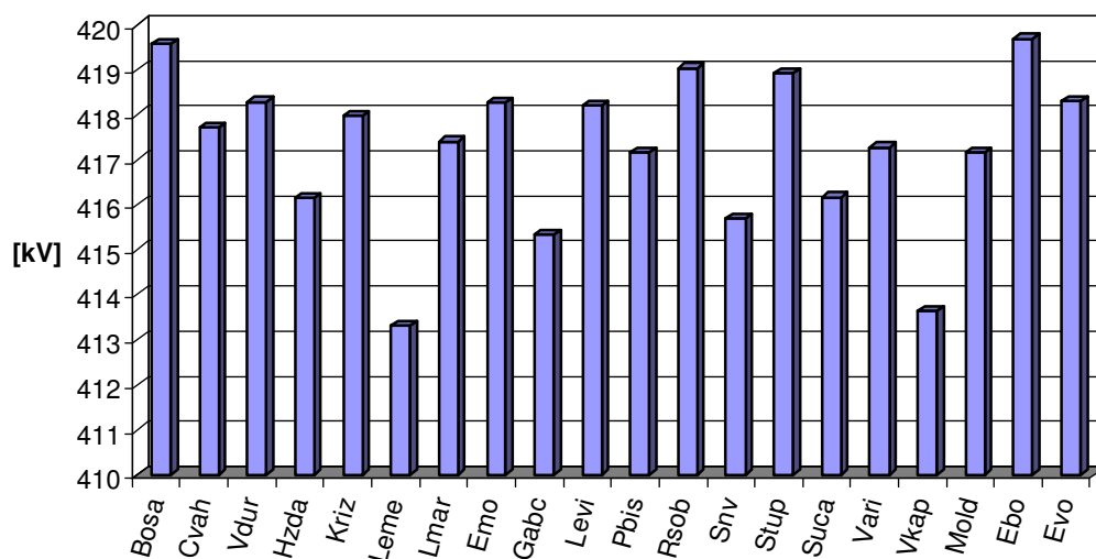
Obr.2. Veľkosť napätia pri výpočtoch letného minima v ES Slovenska
