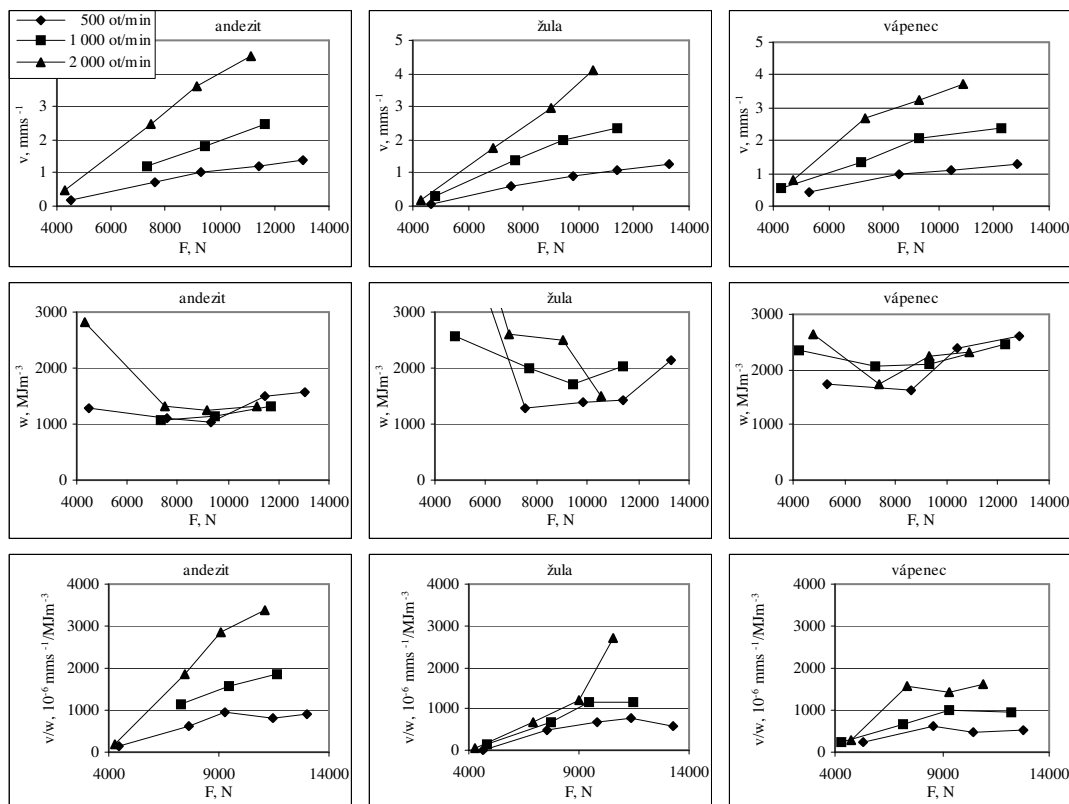
Obr.1: Závislosti rýchlosti vrtania v , mernej objemovej energie rozpojovania w a ich podielu v/w od prítláčnej sily F pre andezit, žulu a vápenec pri troch rôznych otáčkových hladinách
