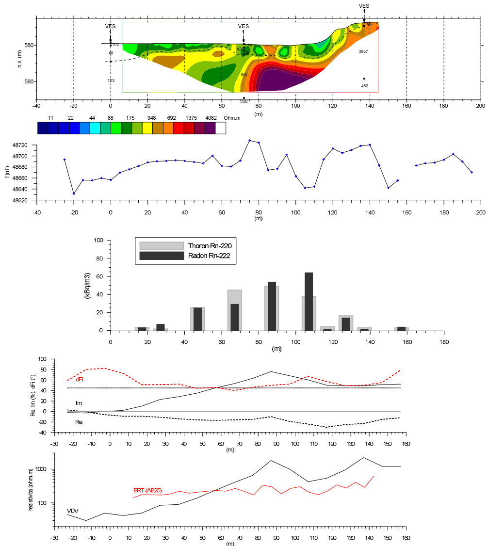
Obr.3: Príklad komplexnej prezentácie výsledkov geofyzikálnych meraní na profile Dielik.
