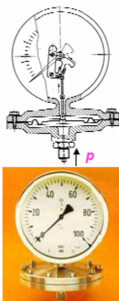
Obr.2.6, Membránový tlakoměr [13]
