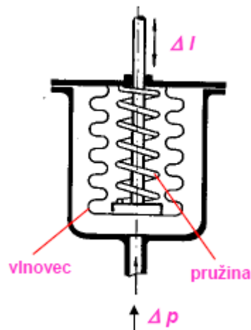
Obr.2.7, Vlnocový tlakoměr [13]
