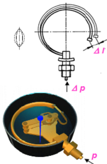
Obr.2.5, Trubicový tlakoměr (Bourdonův) [13]
