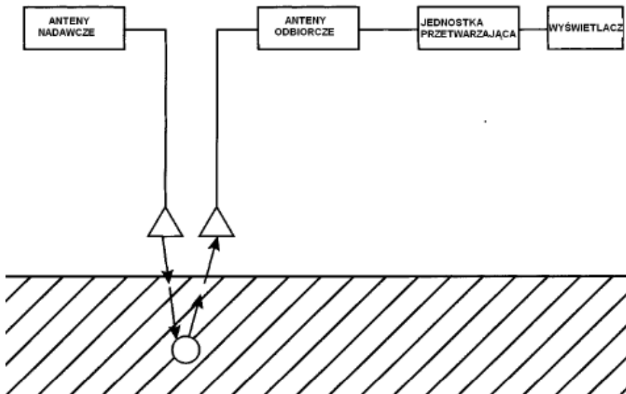
Rys.1 Schemat blokowy radaru GPR
