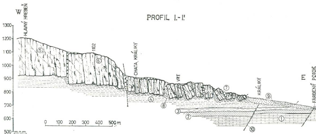
Obr. 2: Charakteristický geologický profil východným okrajom Kremnických vrchov.
