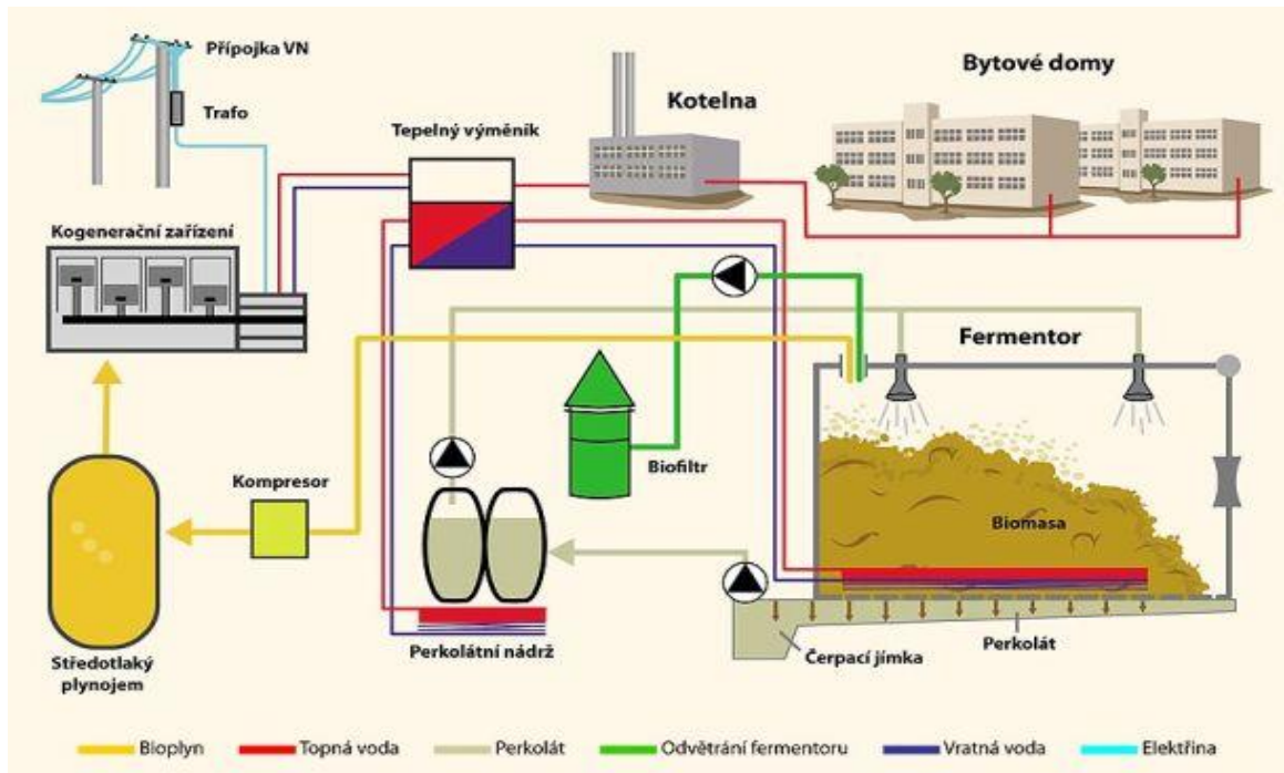
Obrázek č. 18 – Bioplynová stanice – suchá fermentace [7]
