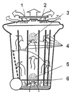
Obrázek č. 8 – Schéma kompostéru [14]
