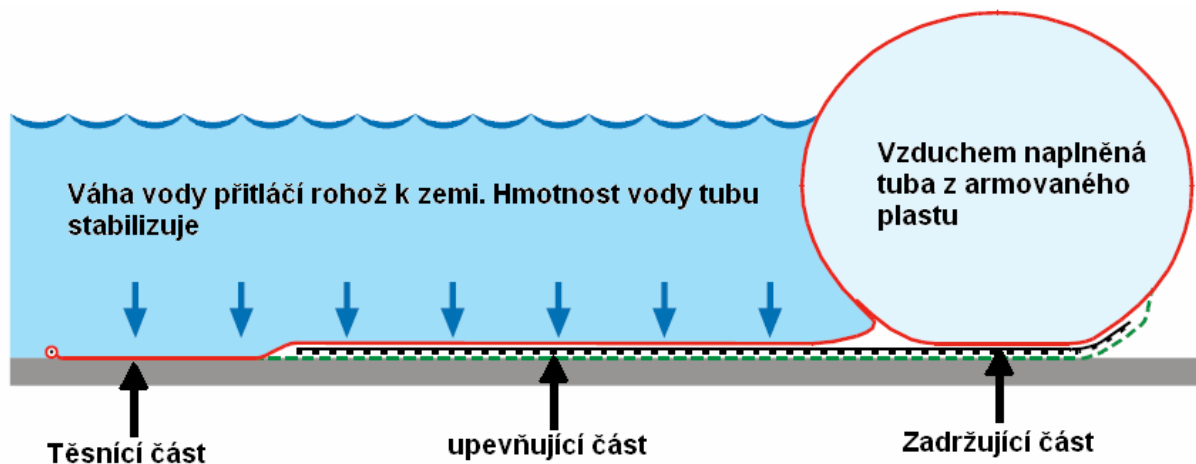
Obrázek 17: NOAQ TW 100 [16]
