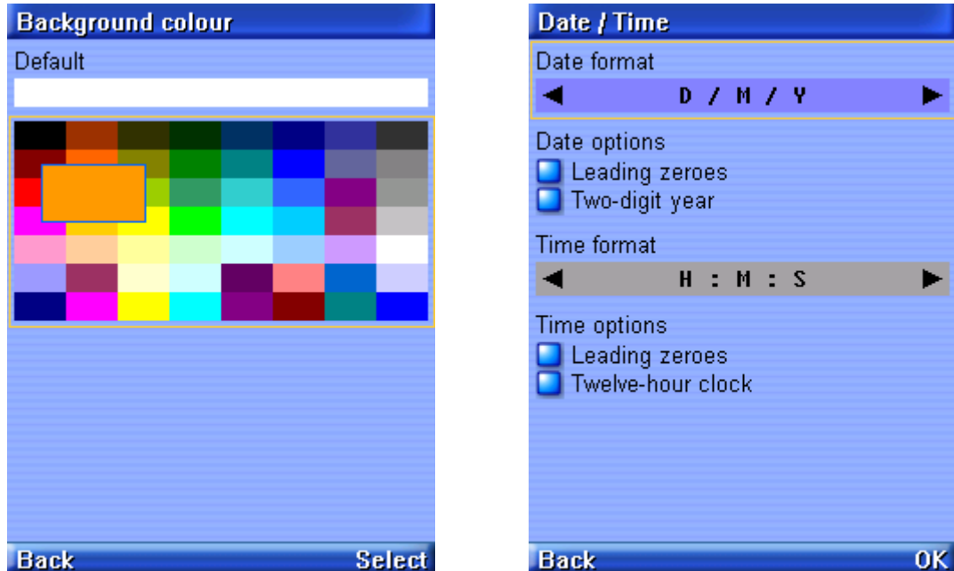
Obrázek 30: Příklad použití komponenty PaletteItem (vlevo) a SelectedItem (vpravo)
