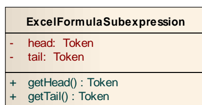
Obrázek 22: Diagram třídy ExcelFormulaSubexpression
