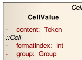
Obrázek 4: Třída CellValue
