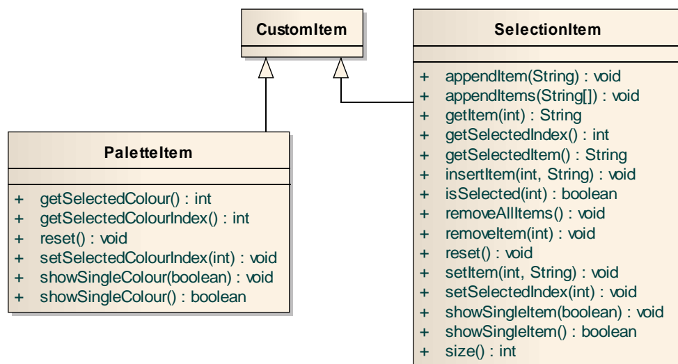
Obrázek 31: Diagram zobrazující hierarchii nových komponent
