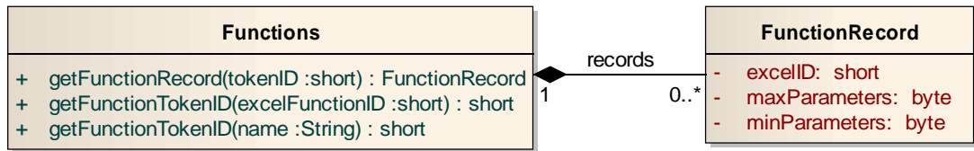
Obrázek 11: Diagram tříd reprezentujících tabulku funkcí
