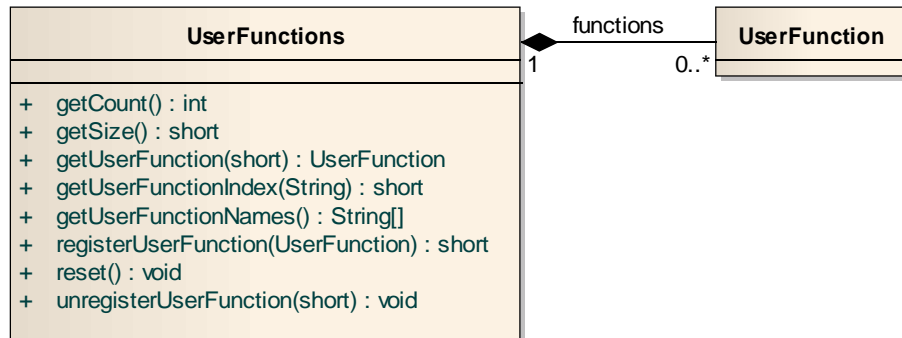
Obrázek 26: Diagram tříd reprezentujících správu uživatelských funkcí
