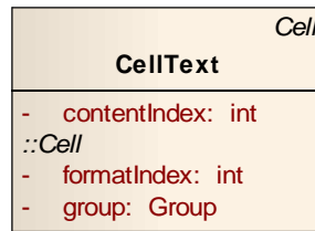
Obrázek 3: Třída CellText
