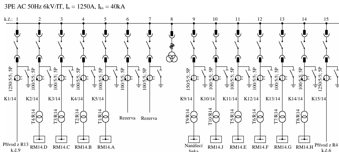
Obř. 16 Jednopolov schma rozvodny R14
