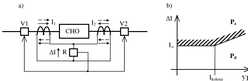
Obr. 9 Rozdílová ochrana:
