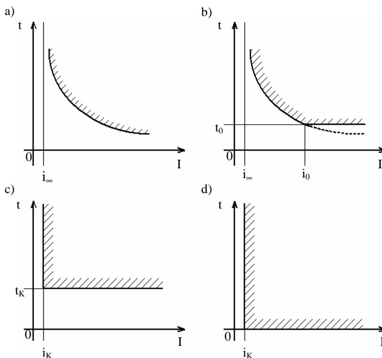
Obr. 5 Charakteristika nadproudových ochran:
