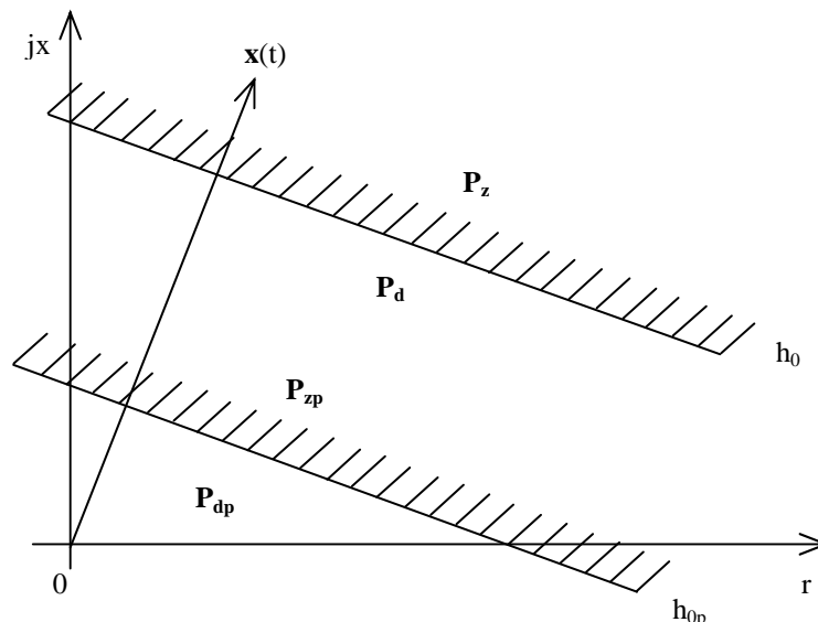
Obr. 3 Charakteristika rozběhového a měřícího členu:
