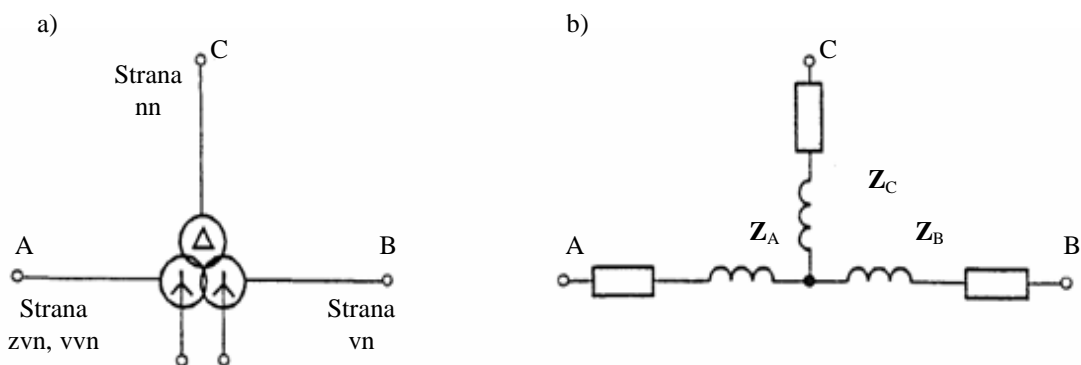
Obr. 14 Trojvinut'ový transformátor:
