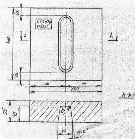
Obr. 5 - Rozměry zkušebního klínu SEW 110 a rozměry uměle vytvořené vady
