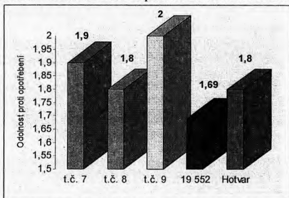
Obr. 5.1 Odolnost proti abrazivnímu opotřebení [ψ a ] jednotlivých zkušebních taveb
